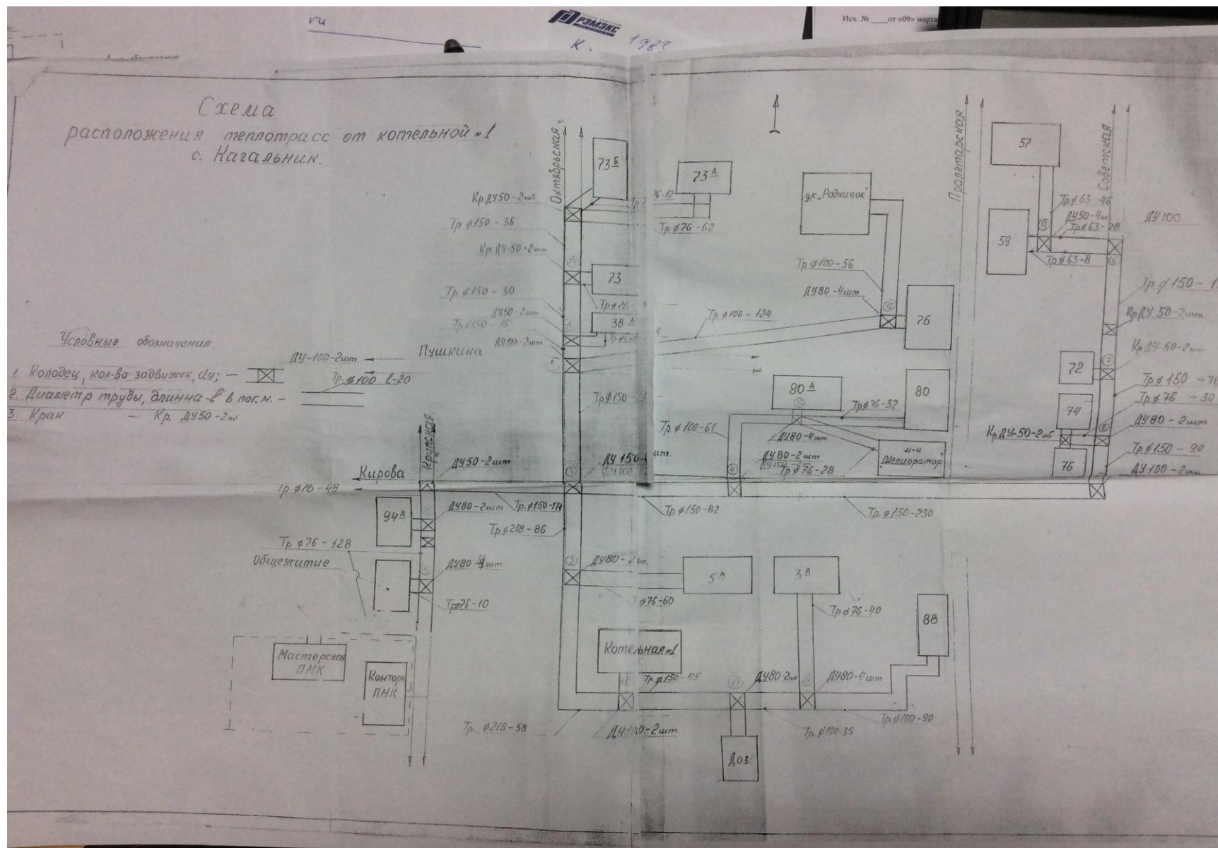
Существующая схема тепловой сети котельной №1
