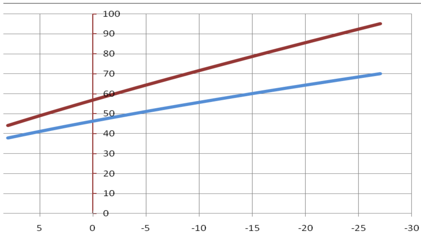
Расчётный температурный график 95/70 °С котельной №1 и №2 с. Кагальник
